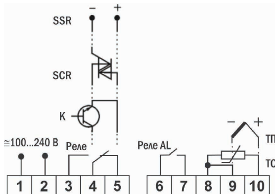
Вид прибора сзади
